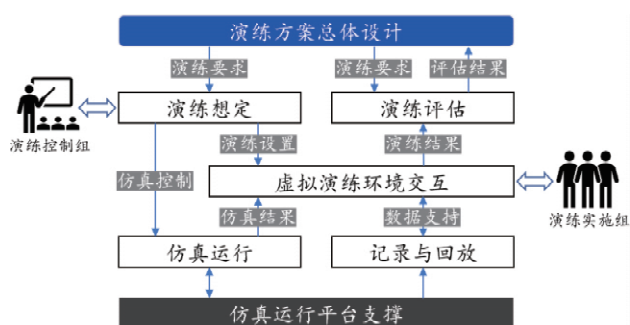
图 2 桌面推演大数据仿真技术框架
