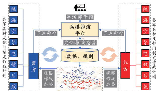
图1 象棋推演流程示例
